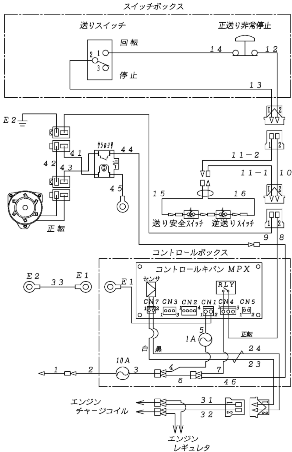
配線図
