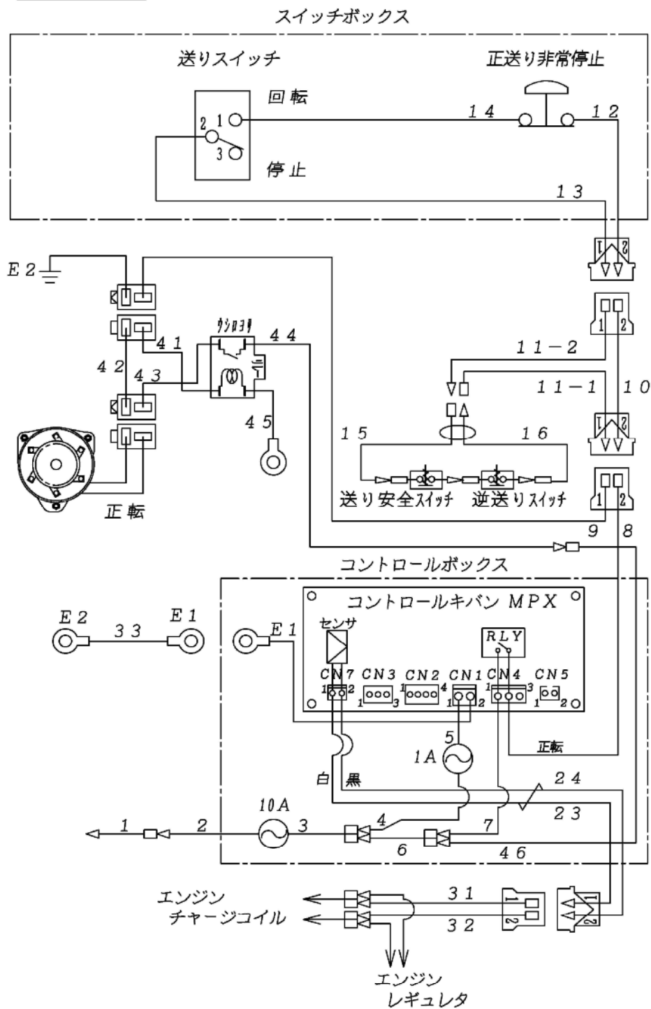
配線図
