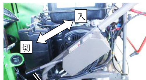
ロータクラッチレバー
