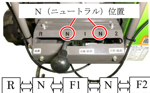
シフトレバー
