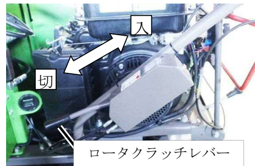
ロータークラッチレバー
