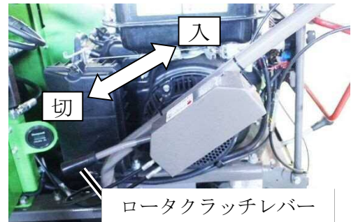
ロータクラッチレバー
