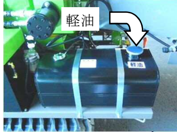
燃料タンク
