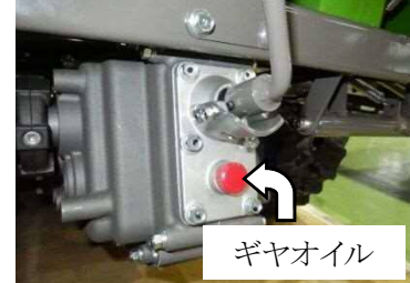
走行ミッション (ホッパー下)
