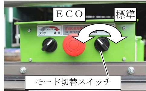
モード切替スイッチ
