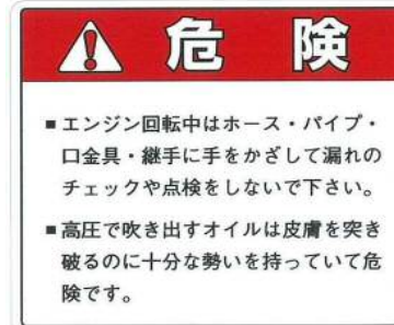
19 油圧ホース
