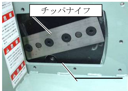
点検窓
