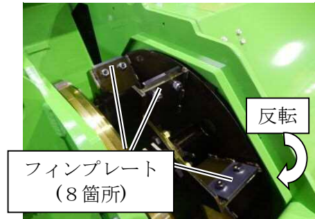
フィンプレート
